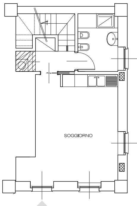
PIANO TERRA (SENZA GIARDINO)
