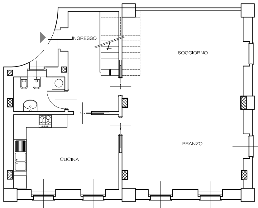
PIANO TERRA (SENZA GIARDINO)
