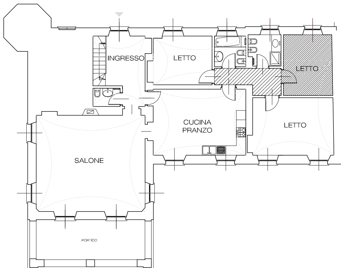
PIANO TERRA (SENZA GIARDINO)
